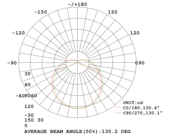
CURVA ISOLUX
